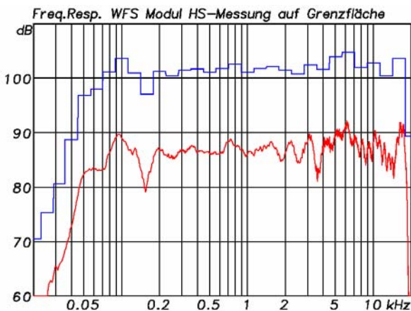
Abbildung 3 Frequenzgang (rot) eines WFS-Kanals innerhalb der Linie auf einer Grenzfläche gemessen. Erreichbarer Maximalpegel in 1 m Entfernung
