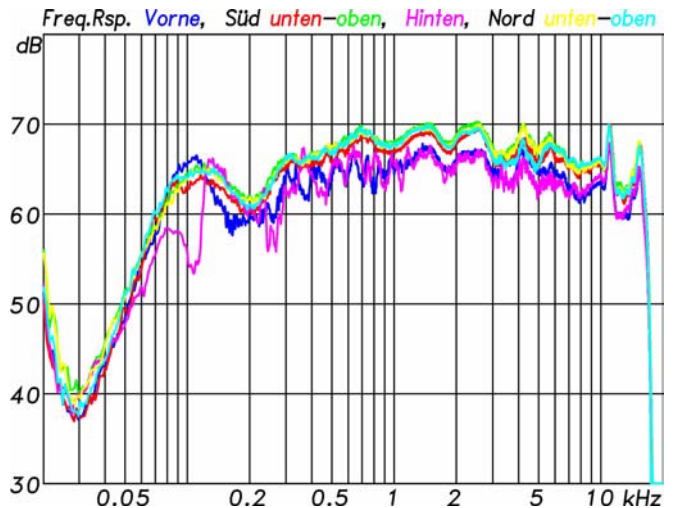
Abbildung 4 Für die sechs Bereiche im Hörsaal gemittelte Frequenzgänge zur Berechnung der EQ-Einstellungen
